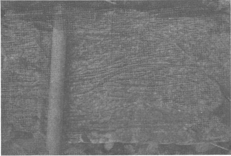
Bild 1: Kleinmaßstäbliche Kreuzschichtung in einer Kalkarenit-Bank. Der Hammerstiel zeigt ins Liegende. Locher Graben 850 m ü. NN, Steinbachtal bei Bihl, Tristelschichten, Zwiesel-Flysch.
