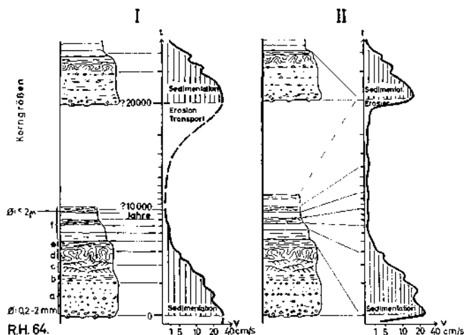
Abb. 1: Graded bedding und Strömungsgeschwindigkeiten a—f: Schichtungsintervalle von Flyschzyklen (modifiziert nach BOUMA 1962). (a) gradiertes Intervall, (b) unteres parallel geschichtetes Intervall, (c) Kreuzschichtungsintervall, (d) Verfälschungsintervall, (e) oberes parallel geschichtetes, z. T. pelitisches Intervall, (f) tonpelitisches Intervall. (I) Sinusförmiger Verlauf der Geschwindigkeitsschwankungen bei normalen Meeresströmungen. (II) Plötzlicher Einsatz hoher Geschwindigkeiten (turbidity currents).
