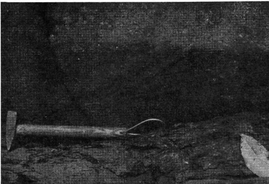
Bild 2: Zwei sich kreuzende Richtungen von Schleifmarken (Winkel = 30^\circ ). Die steilere Richtung durchkreuzt die flachere und ist etwas später entstanden. Jenbachtal bei Feilnbach, 665 m ü. NN, Reiselsberger Sandstein.
